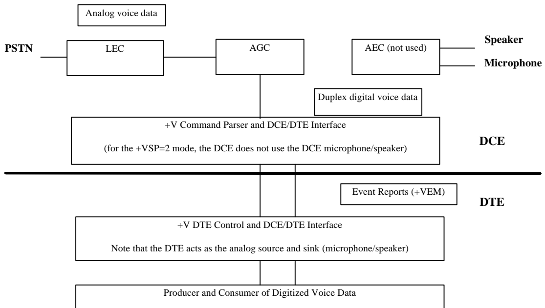
Figure 4 -- PSTN ↔ DTE (+VSP=2)
